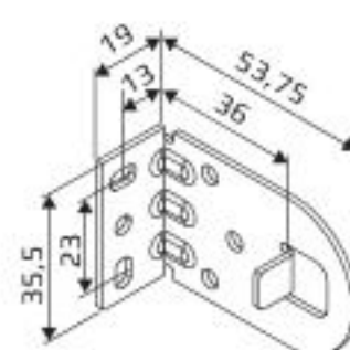
Träger für Sonesse 30 und LS 40
