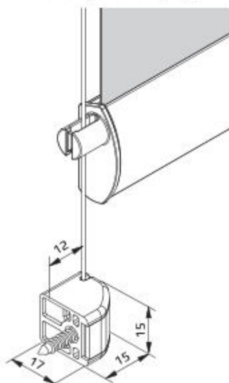
Laibungs-Befestigung
