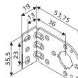
Boden-Befestigung
