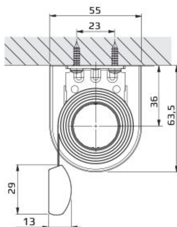
Maße
