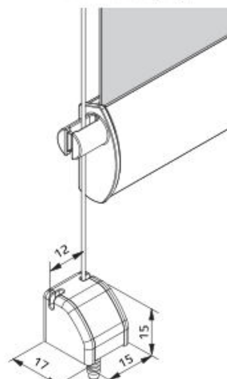
Boden-Befestigung
