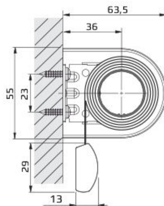
Träger für Sonesse 30 und LS 40
