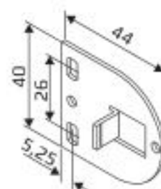
Träger, Laibung (Optional)
