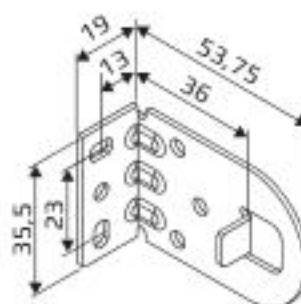
Wand-Befestigung
