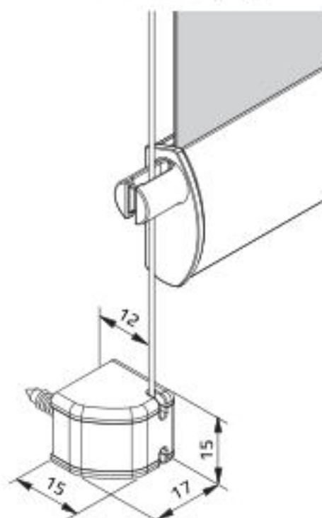
Wand-Befestigung
