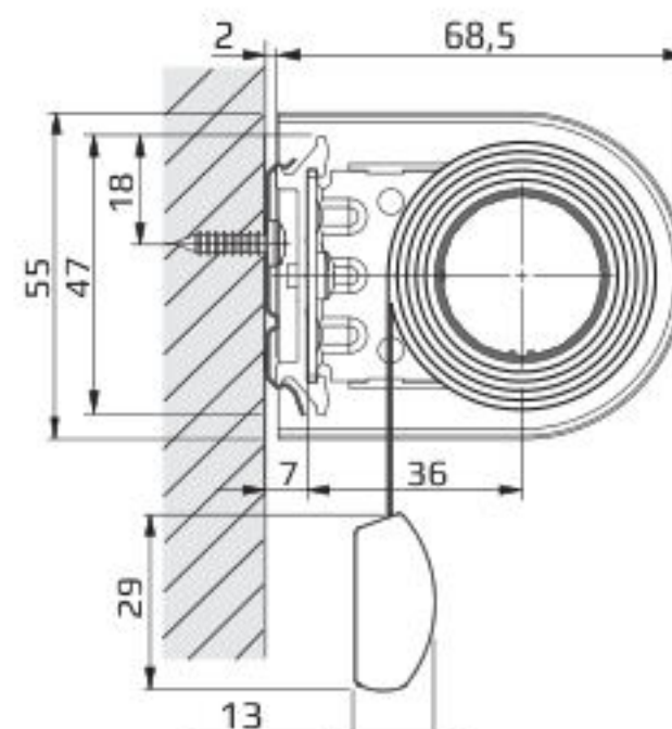
Clip für Trägerprofil
