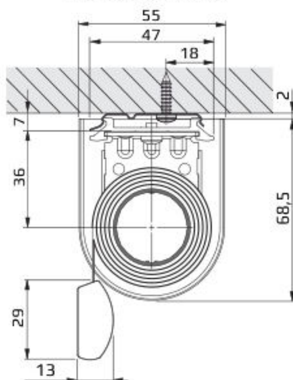
Maße
