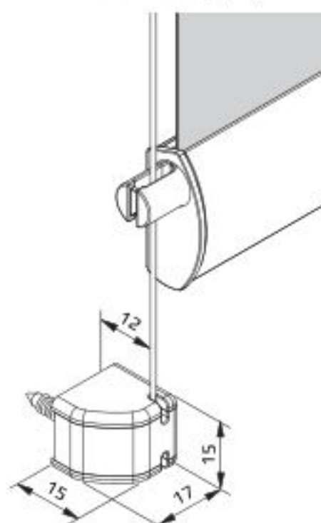
Wand-Befestigung
