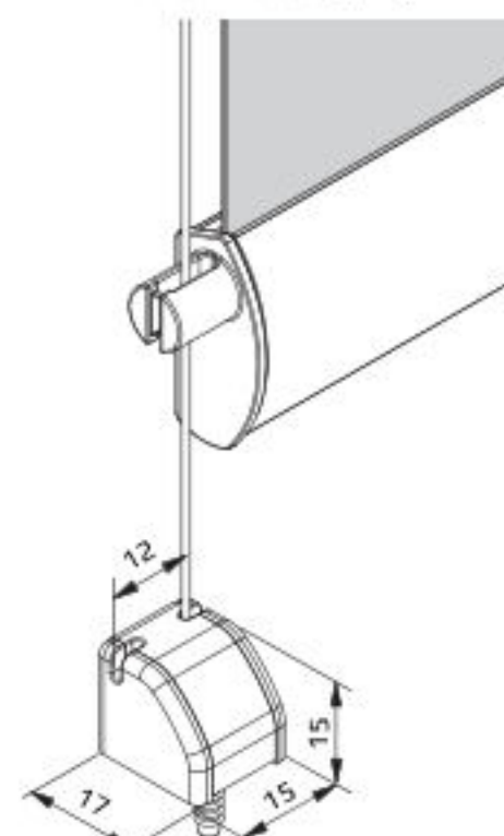
Boden-Befestigung
