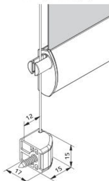
Laibungs-Befestigung
