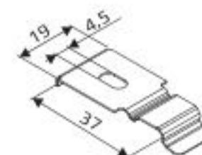
Clip für Kassette und Seitenprofil Montage
