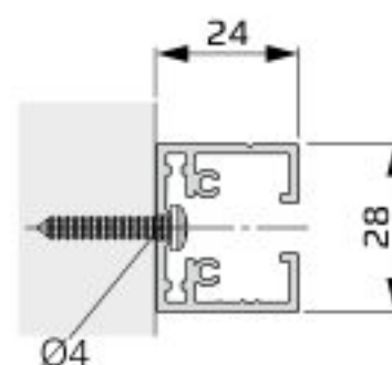
Laibungs-Montage
