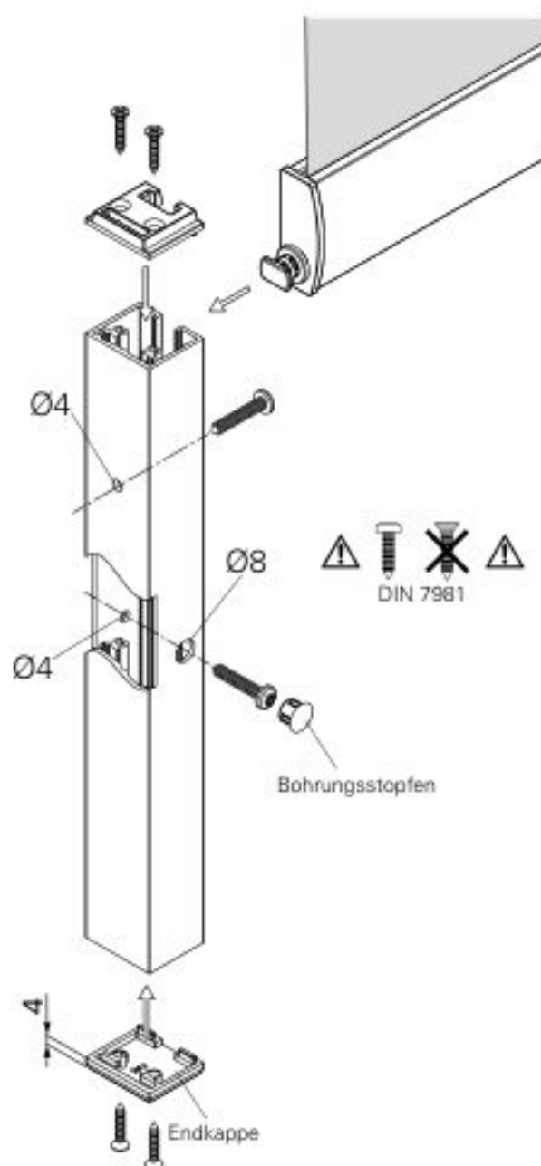
Maße
