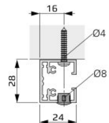
Stirnseitige Montage
