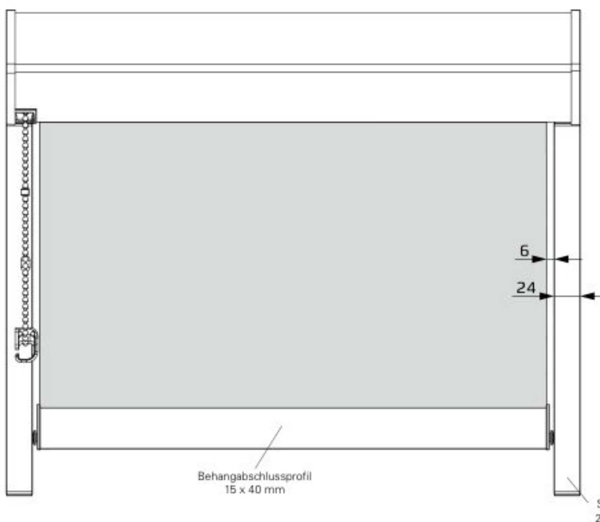
Maße
