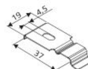
Clip für Trägerprofil
